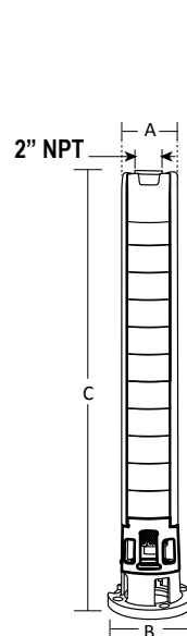
Acoplamiento NEMA 4"
