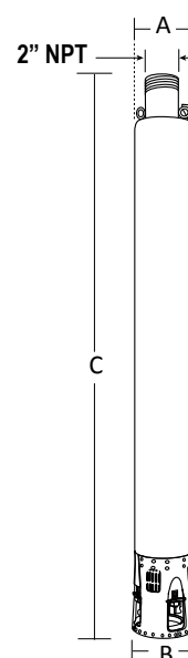
Acoplamiento NEMA 6"
