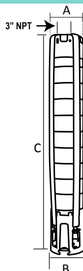
Acoplamiento NEMA 6"
