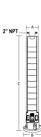
Acoplamiento NEMA 6" Fig. 2
